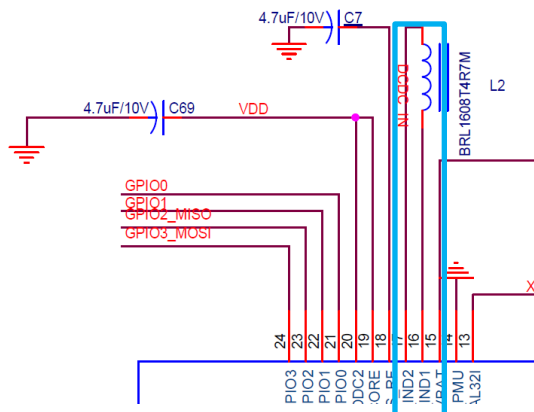
Figure 8. Buck 直流转换器电源电路
